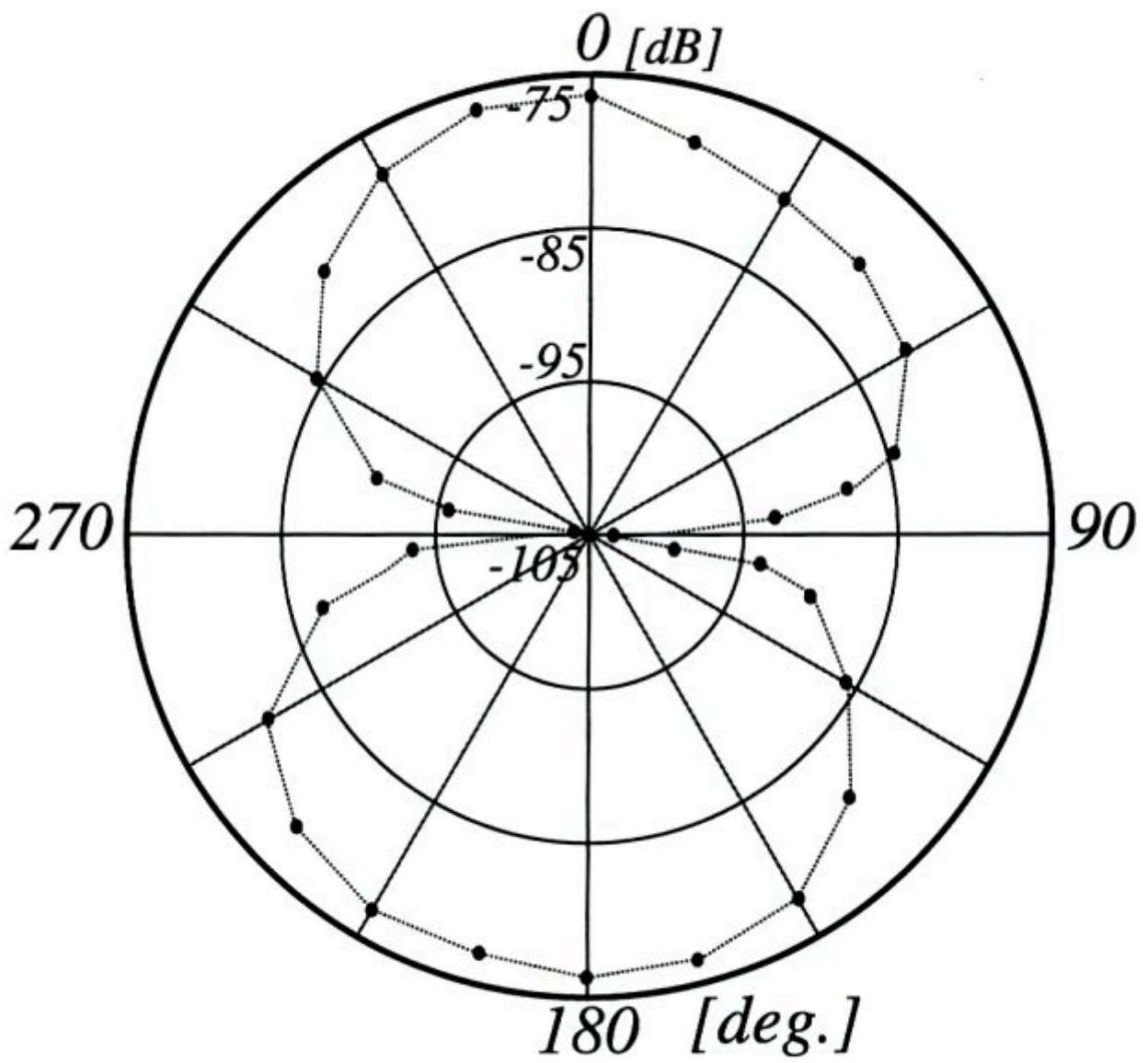
図 3.13: ループアンテナの指向特性 (5 kHz)
