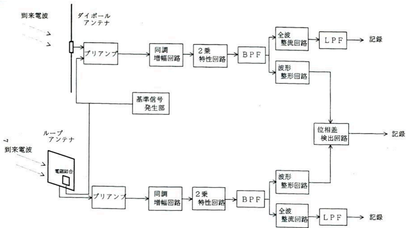
図 2-2-1 観測装置全体のブロック図
