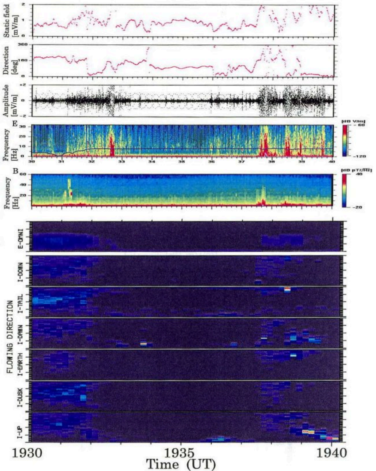
図 4.13 静電場, 静電場の方向, 波動の電界, 波動の電界と磁界の f-t ダイアグラム, 電子とイオンの E-t ダイアグラム
