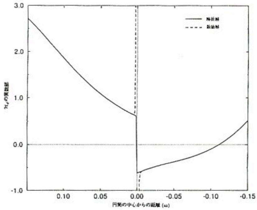
図 G.13 磁界成分の実数部における解析解と数値解の比較
