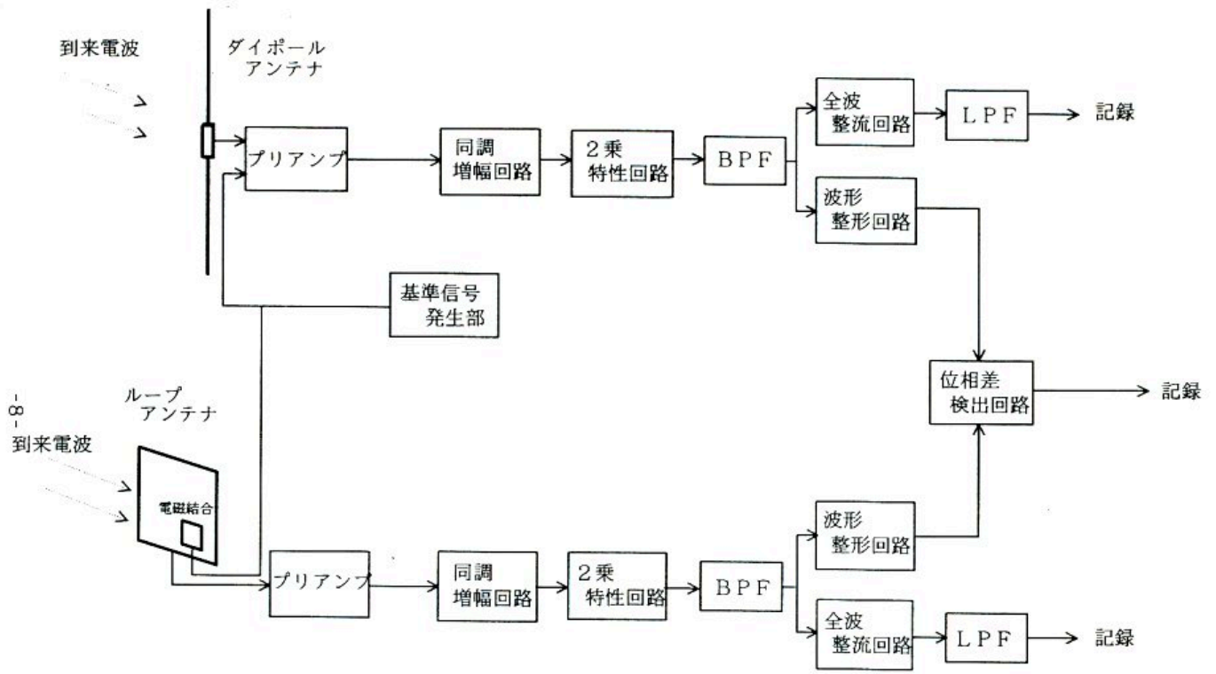
図2-2-1 観測装置のブロック図
