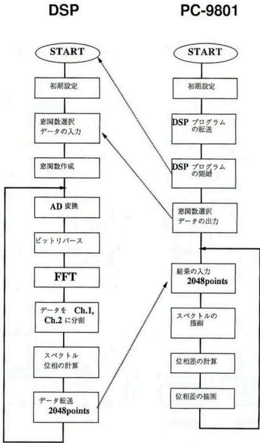
図 4.5 フローチャート
