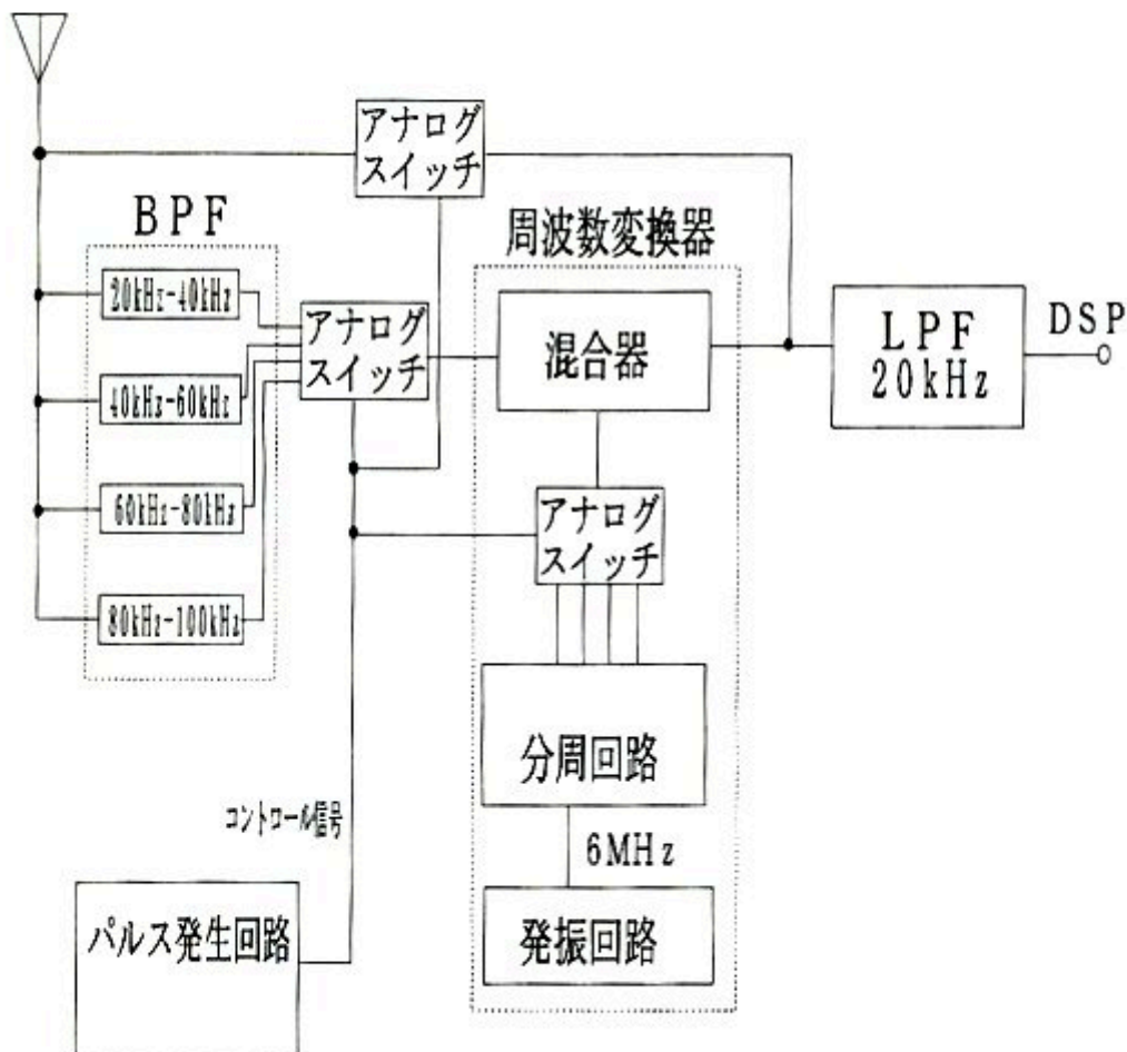
図 1.1 観測装置の概要図
