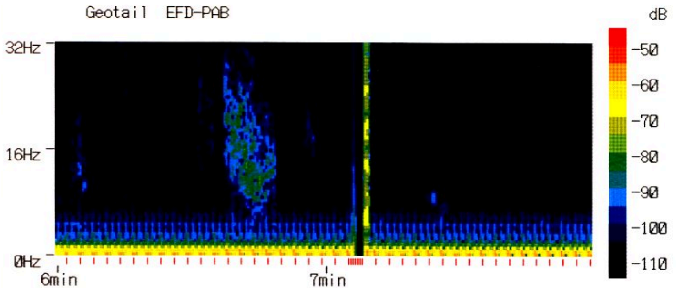
図5-2 1993年10月9日14:06~14:07 UT に観測された波動の電界スペクトル表示
