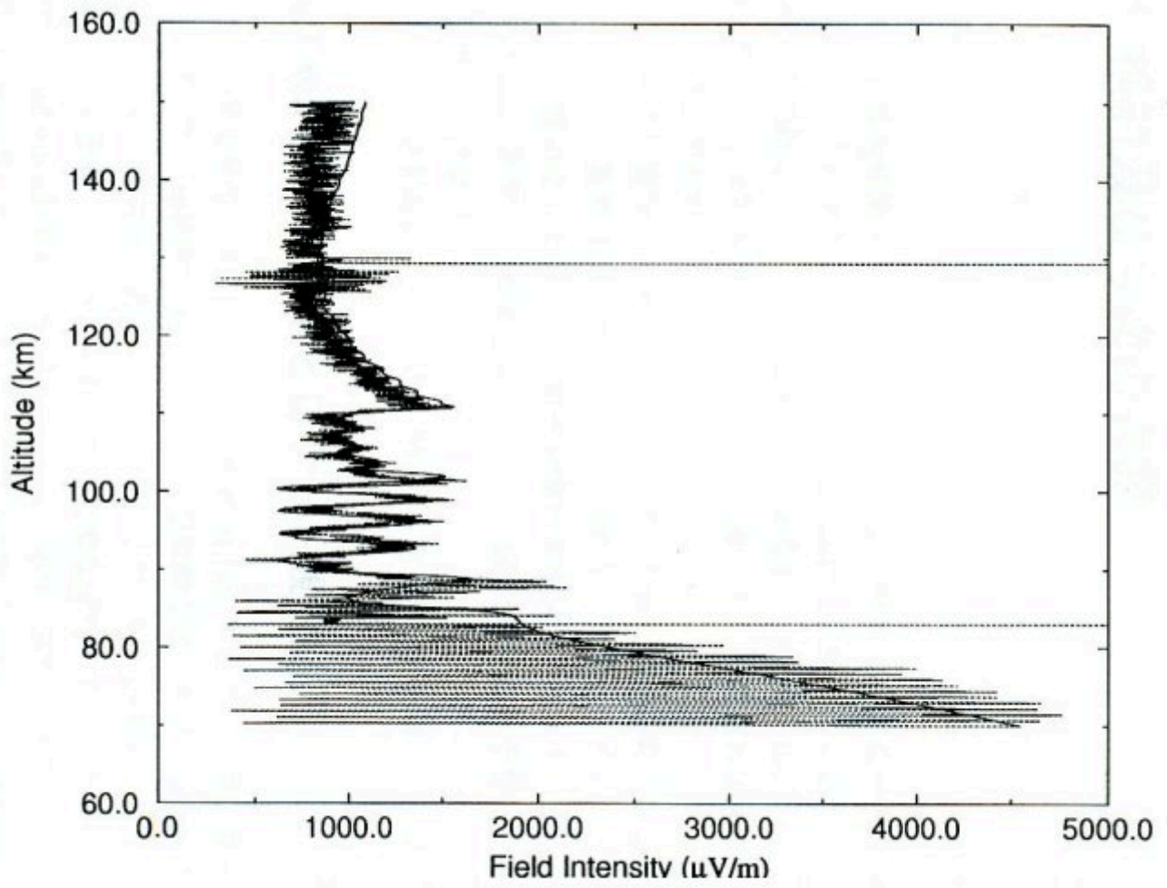
図 4.10 図 4.9 を用いて Full wave 計算して求めた電界強度分布
