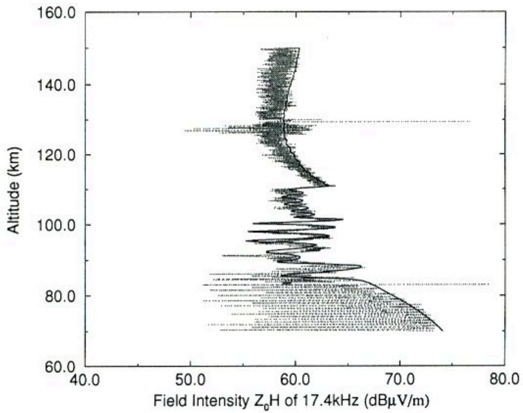
図 4.3 図 4.2を用いて求めた磁界強度分布 実線:Full wave 理論値 点線:ロケット観測値
