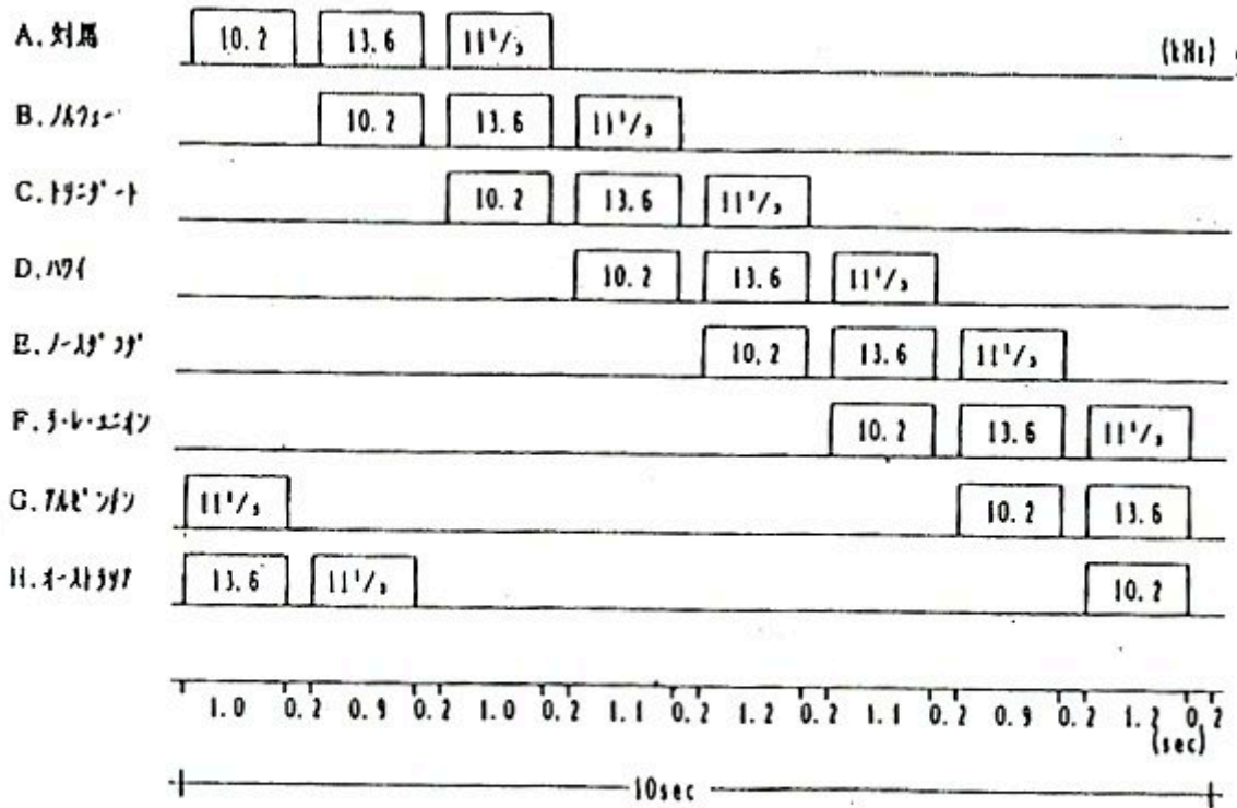
図 1.2 各局の送信パターン
