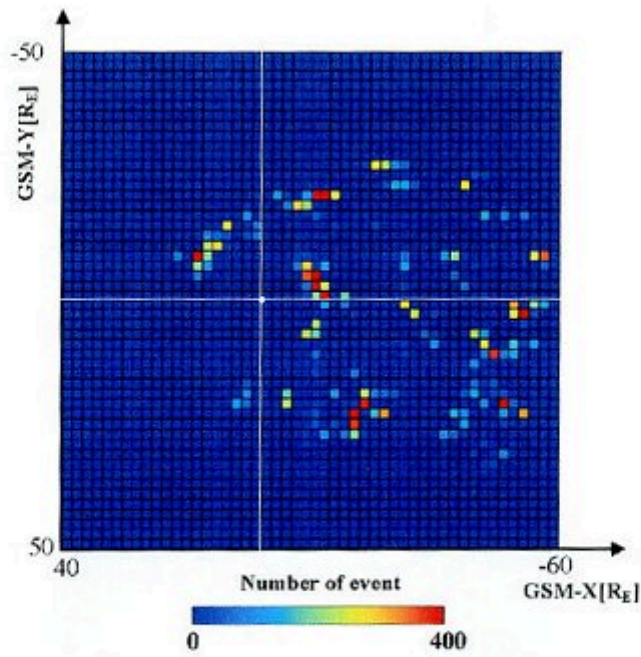
図 3.25: Lobe 領域でのバイポーラ型パルス性波動の X-Y 平面の発生数分布
