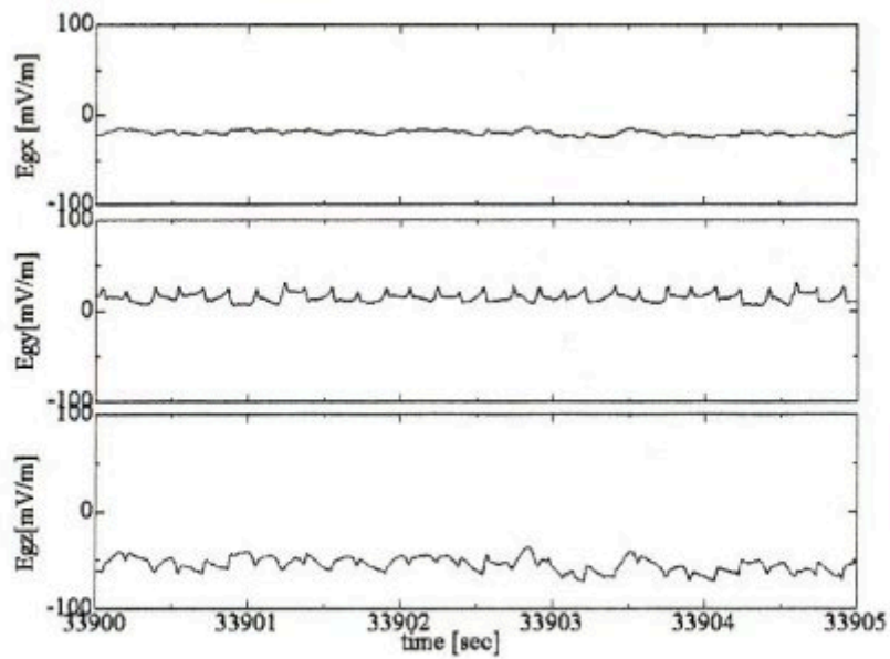
図 4.11: 自然電場を2次元から3次元を計算した波形3成分
