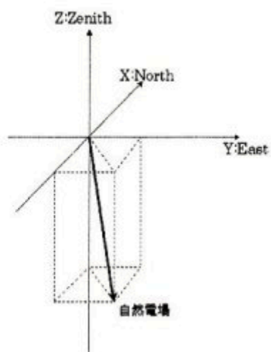
図 4.12: 自然電場の方向の概念図
