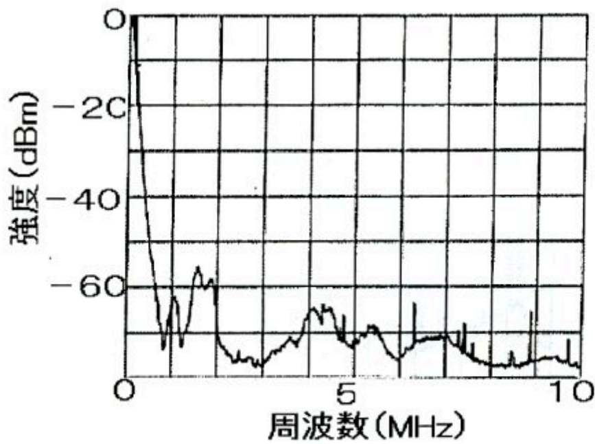
図4.5 各種電気機器からのノイズ(扇風機)
