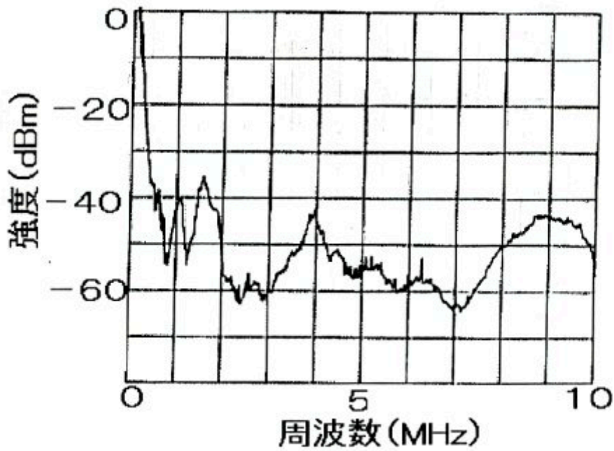
図4.4 各種電気機器からのノイズ(パソコン)
