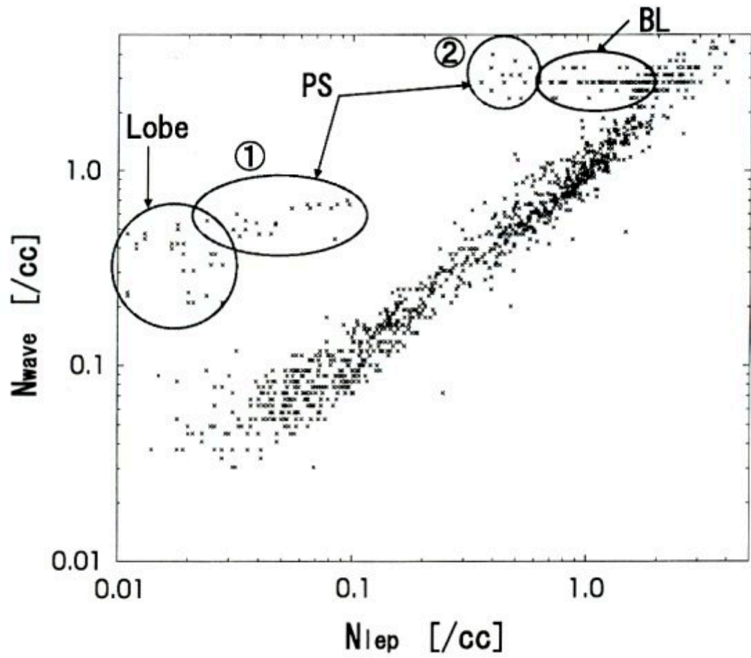
図 3.19: 解析領域全体の N_{lep} - N_{wave} の相関図 (データ数:1100 点)
