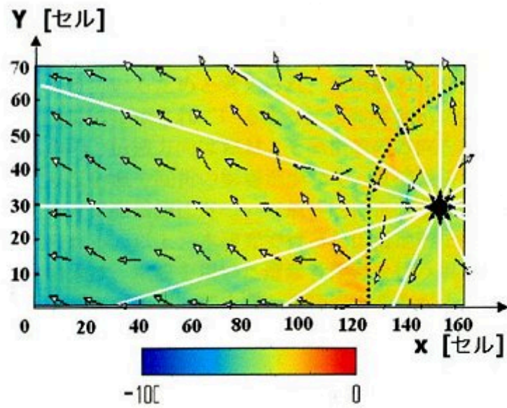
電界強度 [dB V/m]
