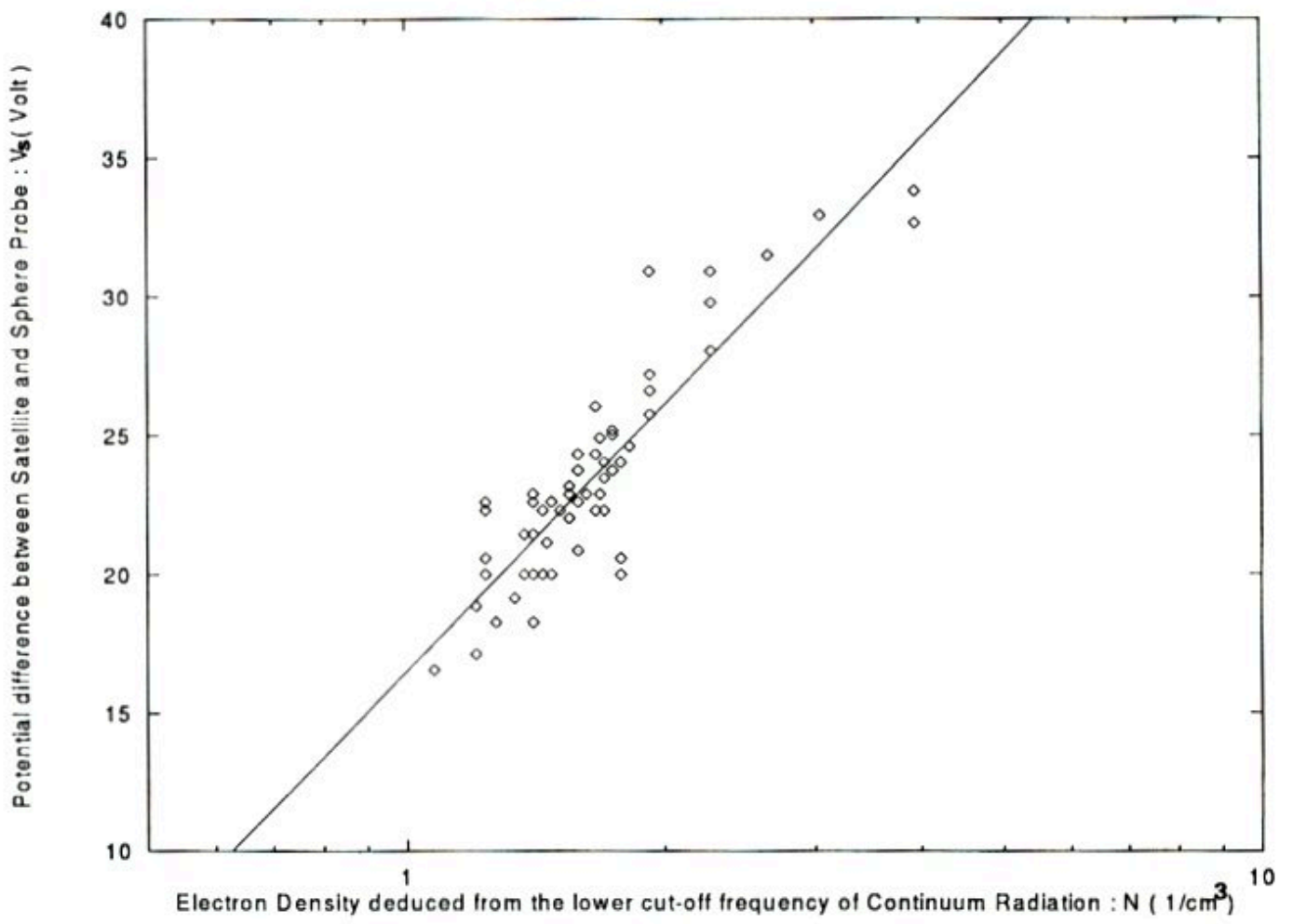
図 7.3 1992 年 10 月 6 日の電子密度と衛星電位の関係
