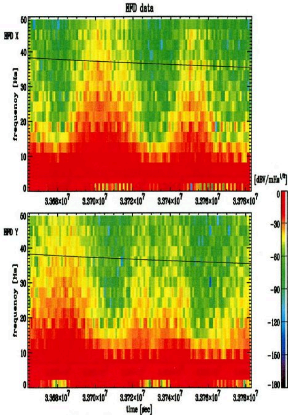
図 A.1 時間 33660～33780 秒間、高度約 791～996km の EFD データの波動表示 (a)は EFD-X、(b)は EFD-Y である。横軸に時間(sec)、縦軸に周波数(Hz)、色の濃淡で電界強度 [\text{dBV/m}\sqrt{\text{Hz}}] を表している
