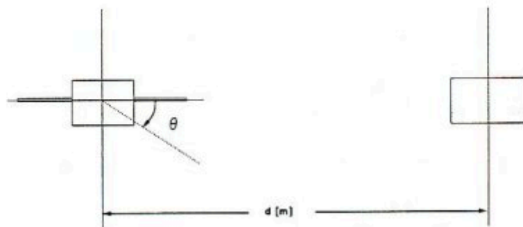
図 5.2 上から見た測定の配置
