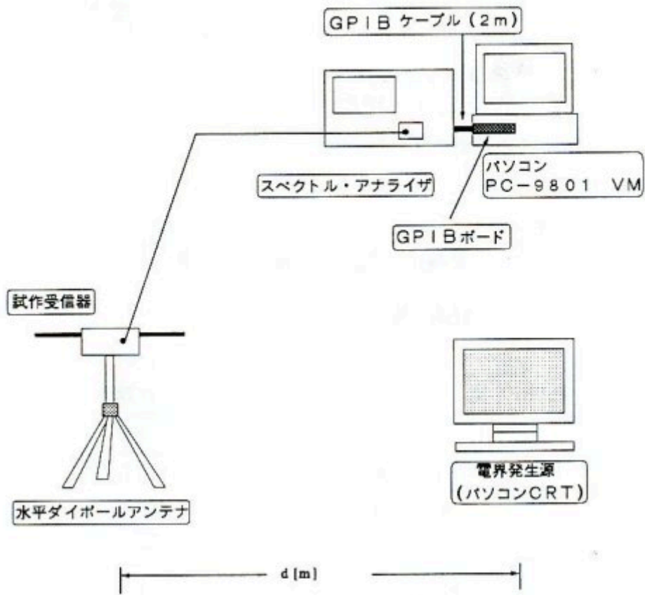
図 5.1 測定機器の接続系統図
