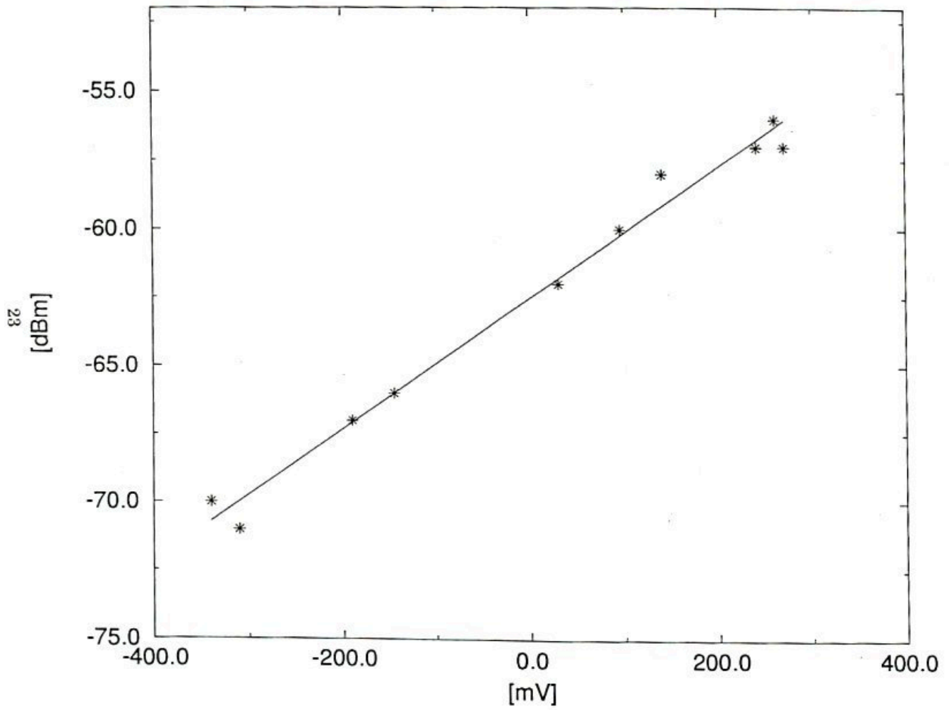
図 4.4 ペンレコーダの値に対するスペクトルアナライザでの信号強度 (CS)
