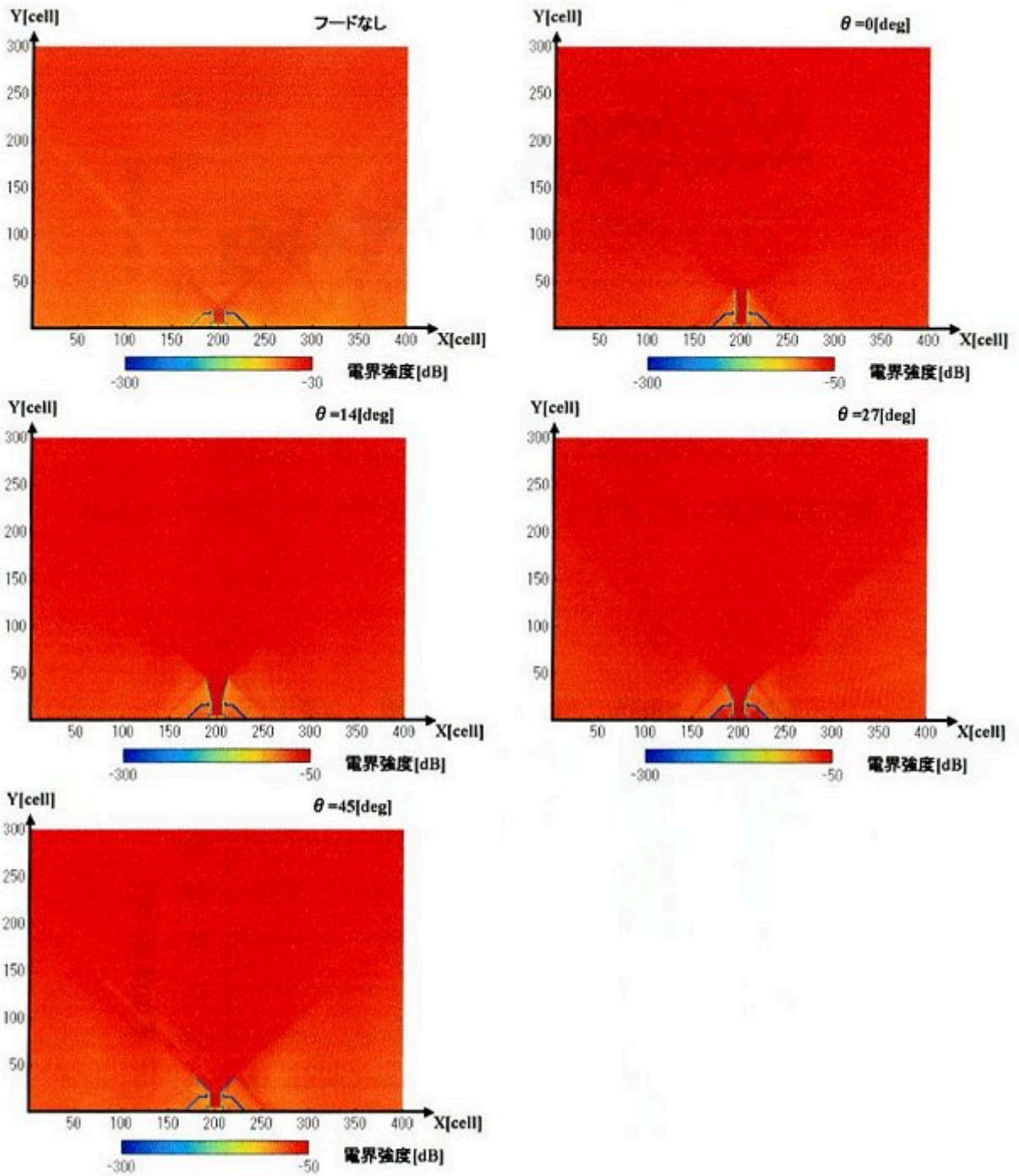
図 4.4: SSC フード角と電界強度分布
