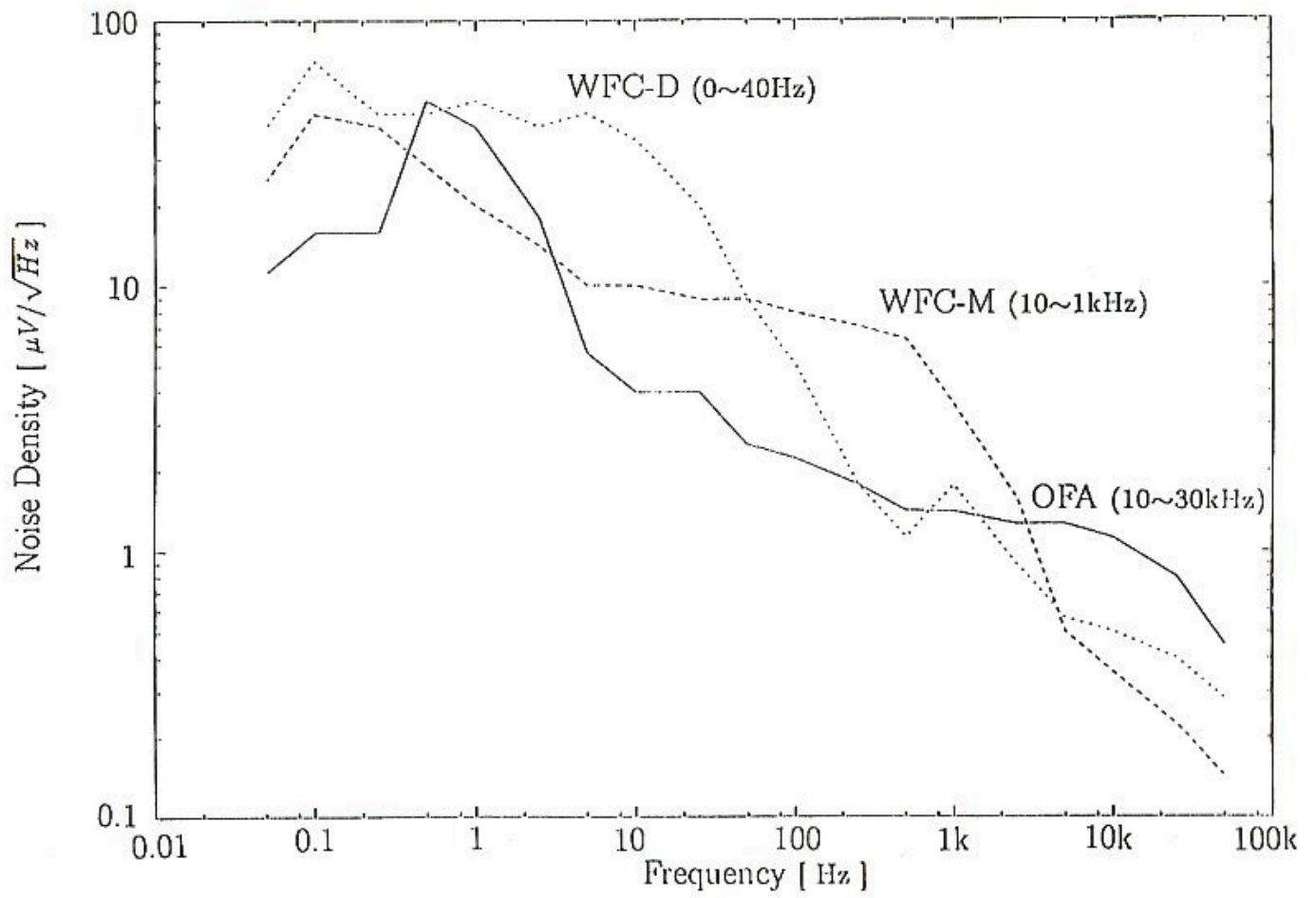
図 4.6 LFA アナログ部の雑音特性
