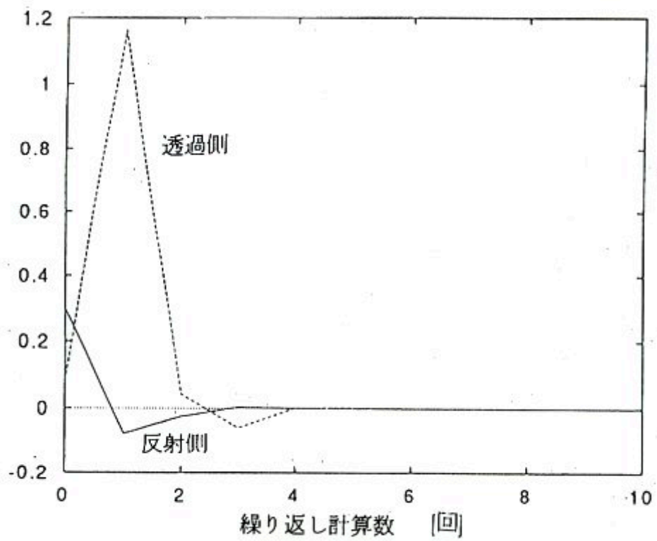
図 4.9 繰り返し計算数と反射側、透過側の位相差の収束分布
