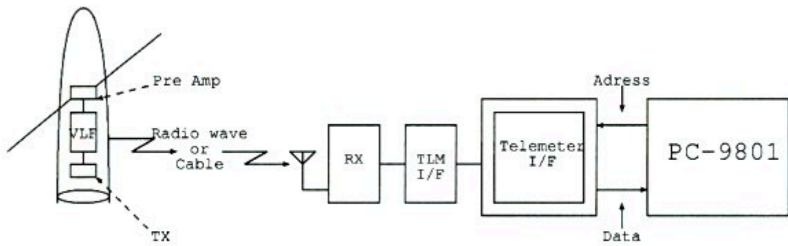
図 4.2 テレメトリ噛み合わせ時の概略図
