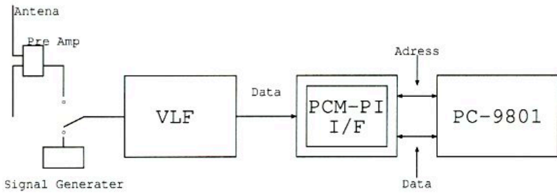
図 4.1 観測装置単体チェック時の概略図
