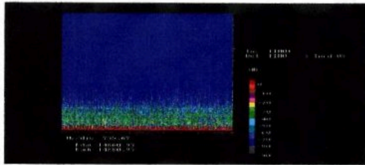
図 5.6 : 扇風機からの距離< 40 c m >
