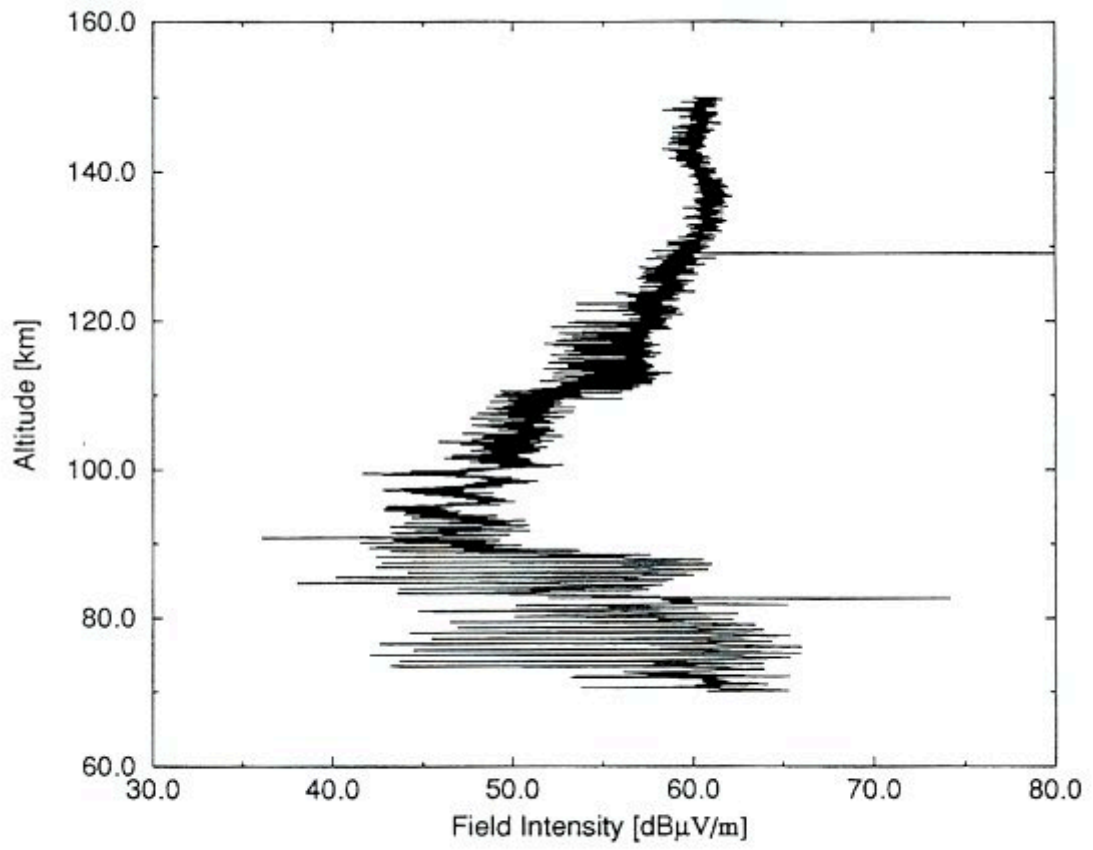
図 4.1 電界強度分布観測データ ループアンテナで観測した VLF 電波の磁界水平成分
