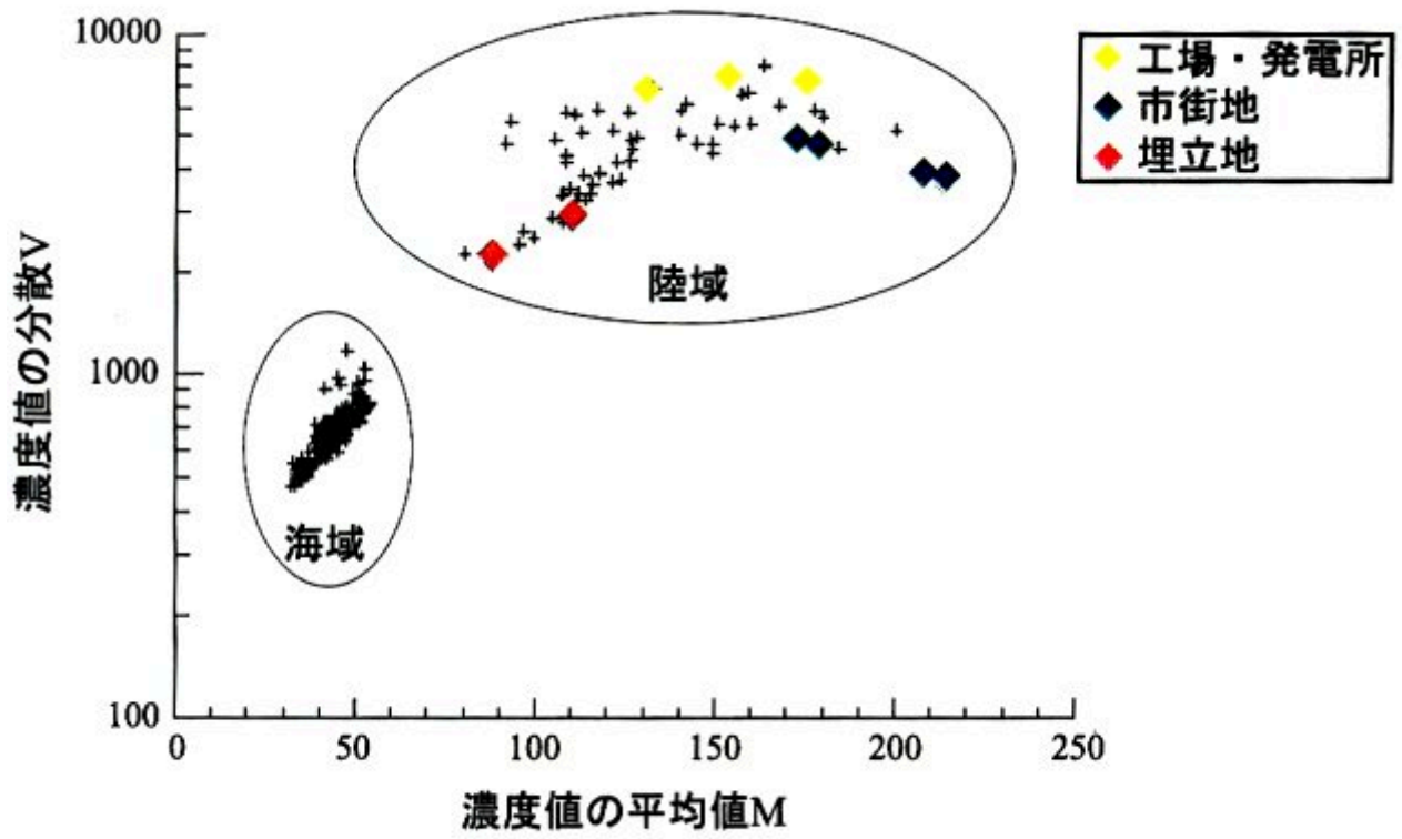
図 4.10: 解析画像全体の後方散乱強度の平均値 M と分散 V の相関
