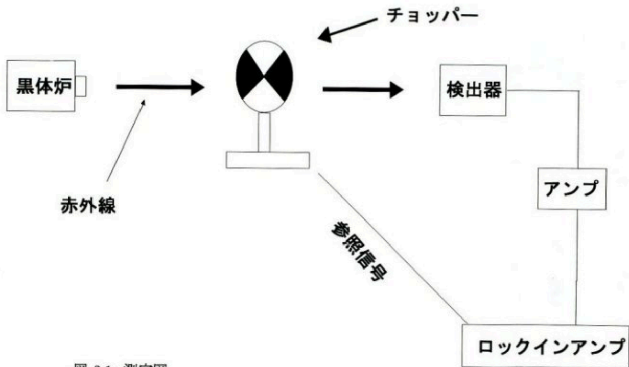
図 3.1: 測定図
